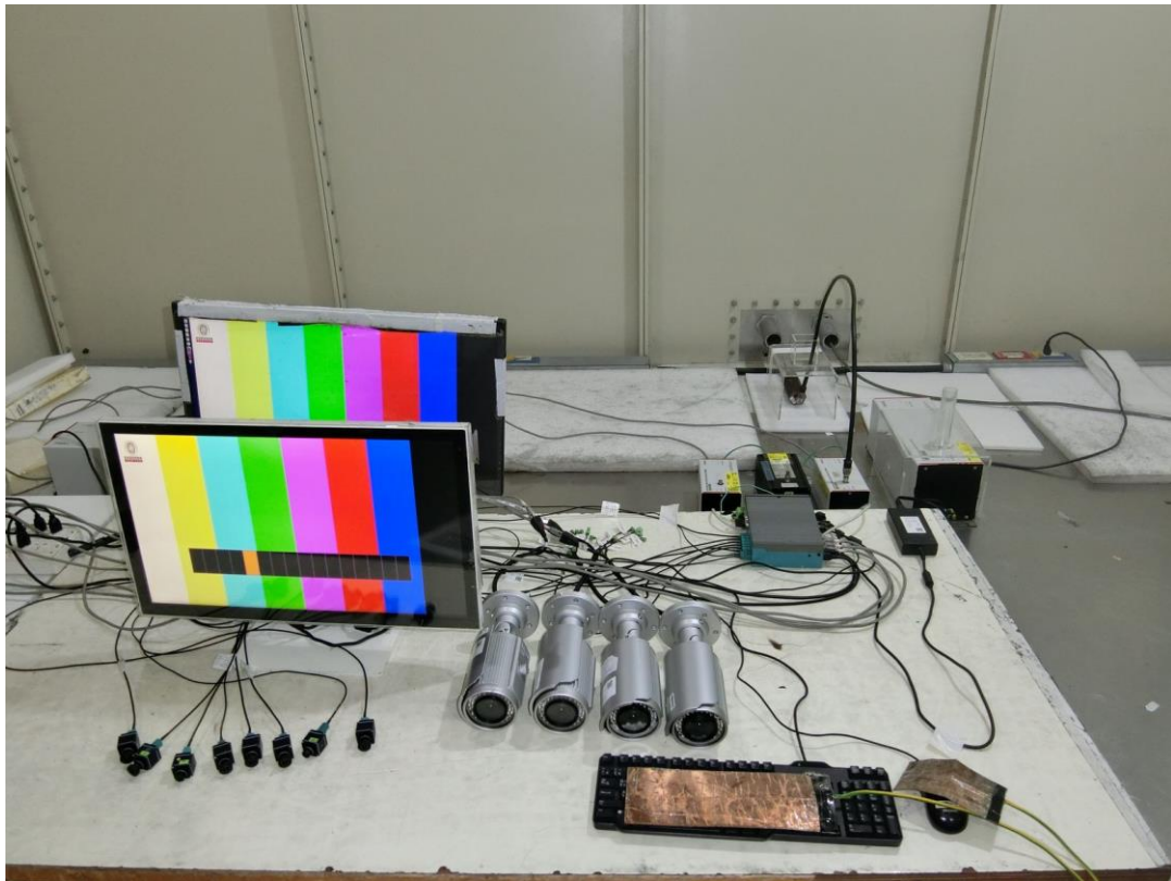
CCD(GMSL1)
