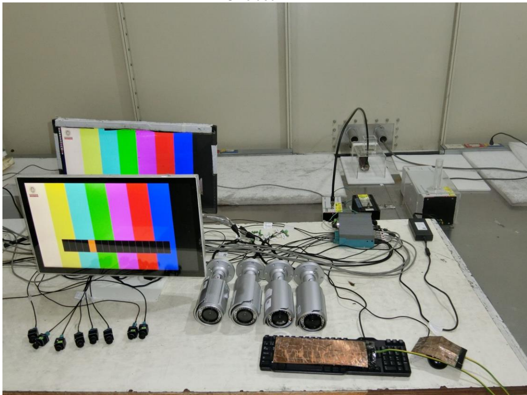
Shielded LAN
