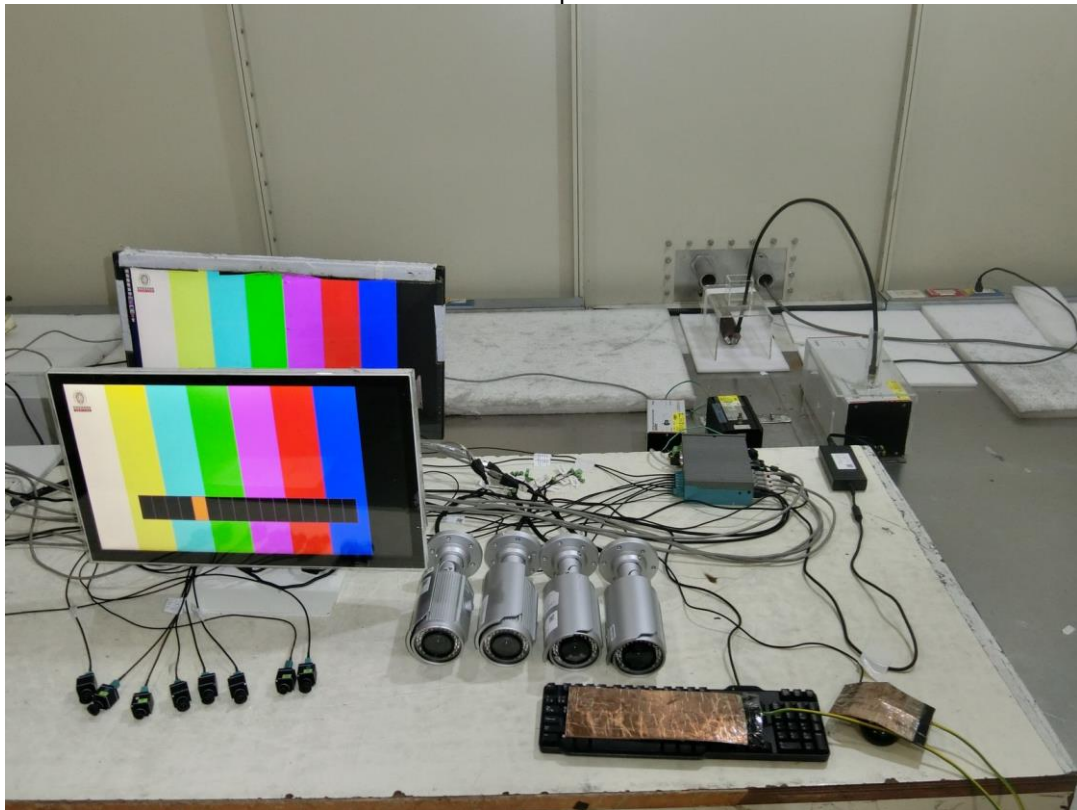
Shielded LAN
